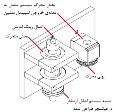
شکل 2 طراحی فیکسچر
