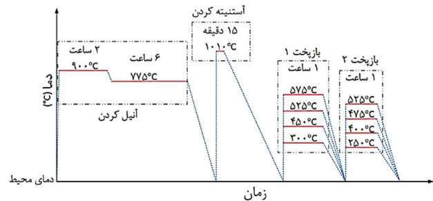
شکل 1 چرخه عملیات حرارتی نمونه‌ها
