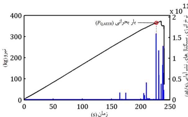
شکل 14 تعیین بار بحرانی به روش نرخ انرژی سیگنال‌های نشر آوایی در نمونه A
