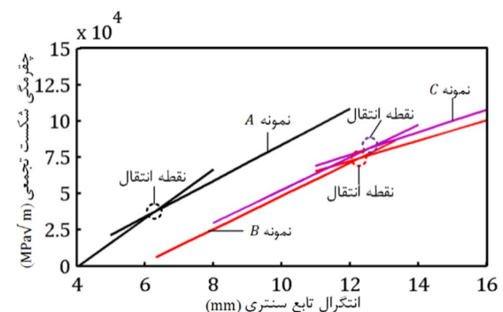
شکل 17 رابطه بین انتگرال تابع سنتری و چقرمگی شکست تجمعی نمونه های A، B و C
