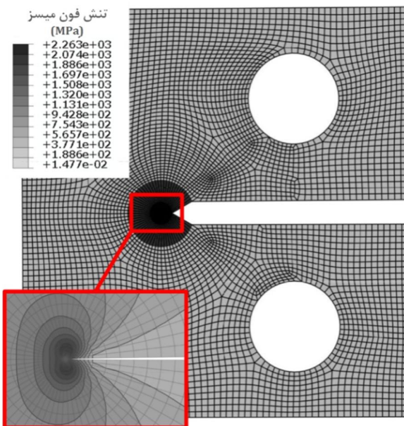
شکل 6 نمونه مدل شده و توزیع تنش فون میسر در نمونه B
