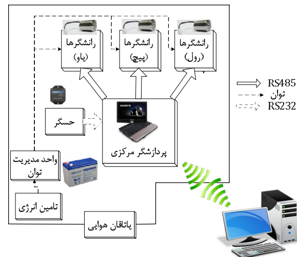
شکل 6 معماری سیستم شبیه‌ساز دینامیک وضعیت 1001
