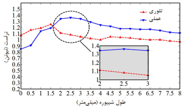
شکل 16 نتایج تست نمونه تحقیقاتی رانشگر گاز سرد
