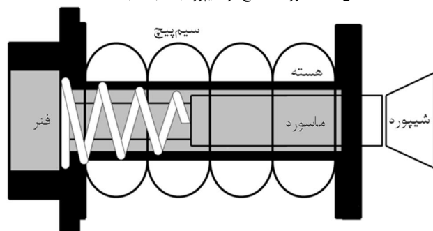
شکل 14 ساختار کلی هر یک از رانشگرهای گاز سرد یکپارچه
