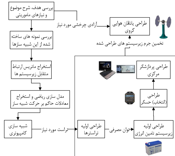
شکل 5 روندنمای طراحی شبیه‌ساز دینامیک وضعیت 1001
