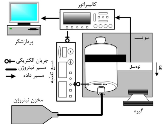
شکل 15 شمای کلی میز اندازه‌گیری تراست
