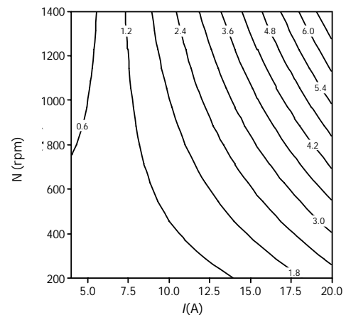
شکل 10 اثر بر هم کنش متغیر جریان و سرعت دوران الکتروند
