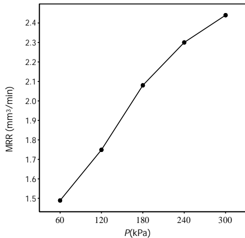
شکل 15 اثر فاکتور اصلی فشار گاز ورودی بر نرخ باربرداری
