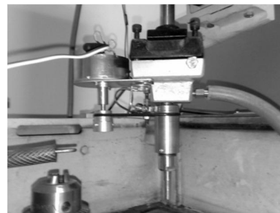
شکل 3 دستگاه ماشین کاری تخلیه الکتریکی خشک
