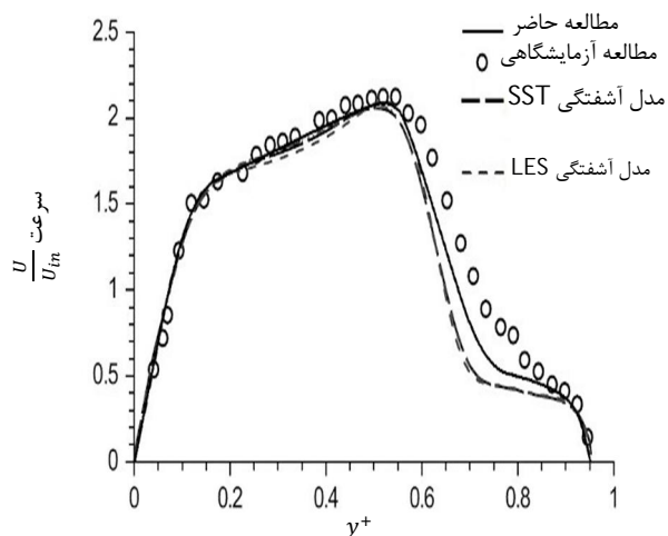
شکل 4 مقایسه مطالعه حاضر با مدل های آشفنگی انتقال تنش برشی و شبیه سازی گردابه های بزرگ و همچنین کار آزمایشگاهی
