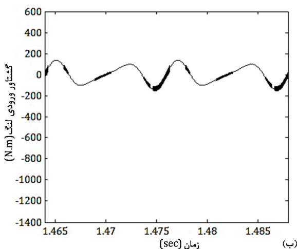
شکل 7 منحنی گشتاور ورودی به ازای دو دوران کامل لنگ، (الف) مدل تماس خشک، (ب) مدل روانکاری شده
