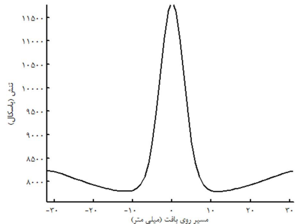
شکل 4 نمودار تنش لامسه ای اندازه گیری شده در سطح بافت نرم مافوق الاستیک
