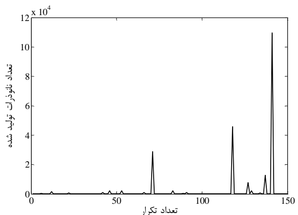
شکل 2 تعداد نانوذرات تولید شده برای نانوسیال آب-اکسید آلومینیم (15 نانومتر) با 1 درصد حجمی در 150 بار اجرای برنامه
