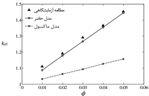
شکل 8 مقایسه مقادیر ضریب هدایت حرارتی مؤثر با داده‌های آزمایشگاهی ایستمن [3] و نتایج سایر مدل‌ها برای نانوسیال اتیلن گلیکول - آلومینیوم با قطر متوسط 36 نانومتر
