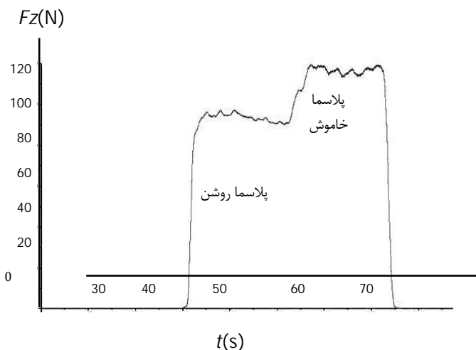
شکل 8 اندازه‌گیری نیروی اصلی تراش هنگام تراش کاری به کمک پلاسمای
