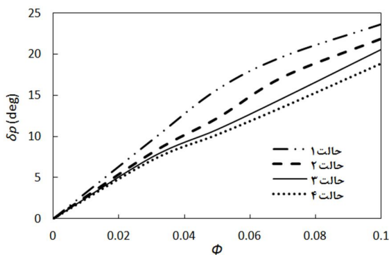
شکل 13 مقایسه زاویه برداردهی (درجه) بدست آمده با شیارهای مختلف
