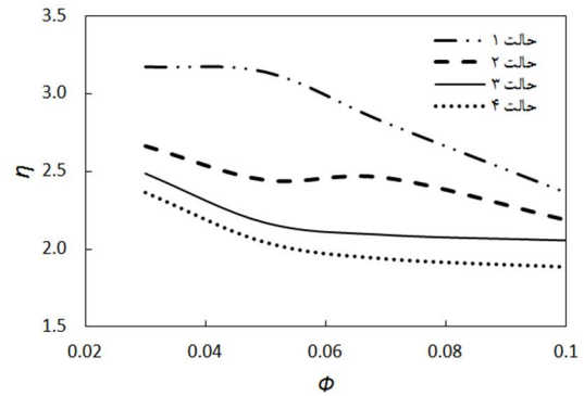
شکل 14 مقایسه بازدهی برداردهی بدست آمده با شیارهای مختلف
