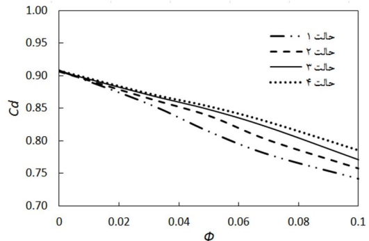
شکل 10 مقایسه ضریب تخلیه بدست آمده با شیارهای مختلف
