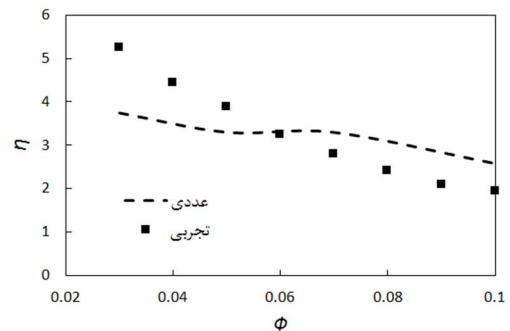
شکل 7 مقایسه نتایج عددی و تجربی برای بازدهی برداردهی
