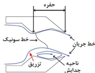
شکل ۱ نمایش عملکرد نازل‌های DTN و تزریق جریان ثانویه [1]
