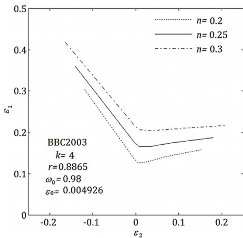
شکل 17 اثر توان کرنش سختی بر FLD براساس مدل MK و معیار تسلیم BBC2003
