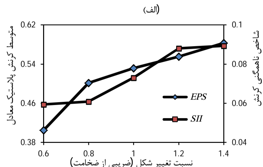
شکل 10 الف- اثر نسبت تغییر شکل بر روی توزیع کرنش پلاستیک ب- اثر نسبت تغییر شکل بر روی متوسط کرنش پلاستیک و شاخص ناهمگنی کرنش
