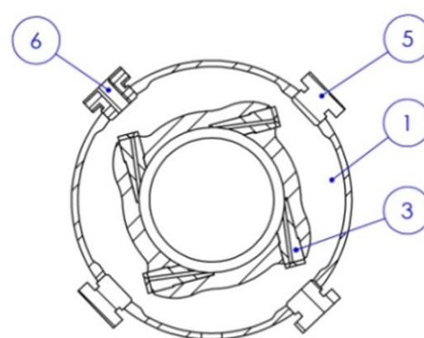
شکل 4 شمایی از طرح محفظه به منظور تست سرد 1 و 7- کالکتور سیال؛ 2- محفظه پلکسی گلس؛ 3- انژکتور مماسی؛ 4- پله‌ی تکیه‌گاهی؛ 5- منفذ ورودی جهت تعویض انژکتورها؛ 6- ورودی سیال
