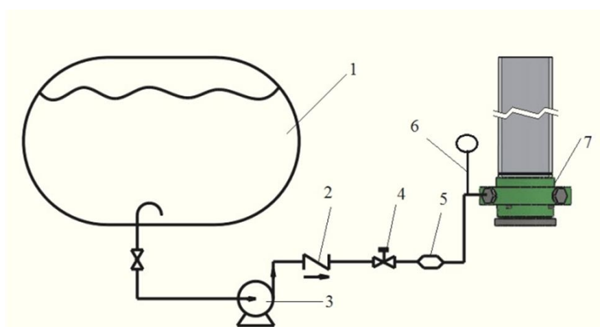
شکل 7 شمایی از مدار تست
