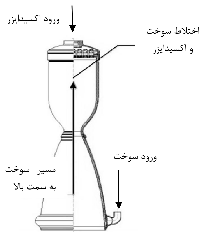
شکل 1 شماتیکی از محفظه احتراق جریان محوری [2]
