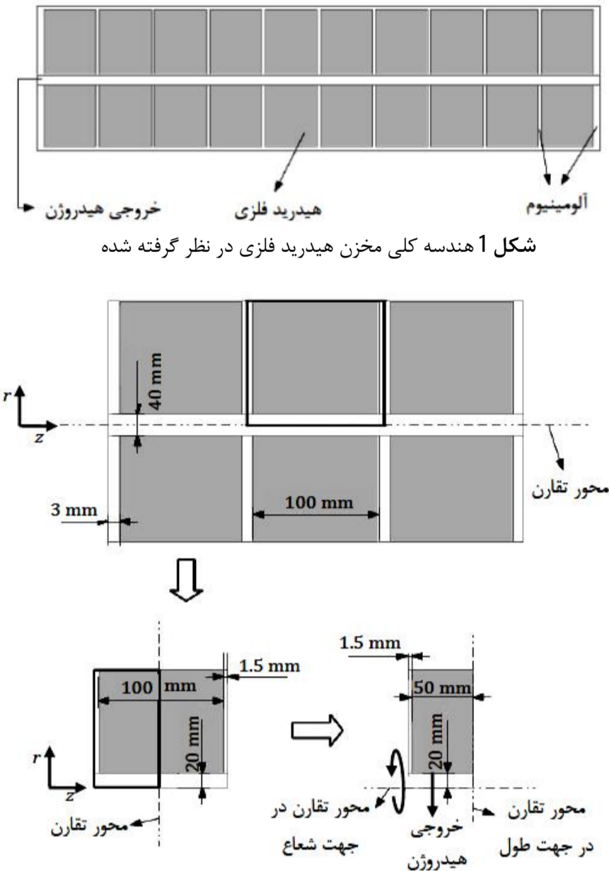
شکل 2 ابعاد و نحوه انتخاب هندسه شبیه‌سازی
