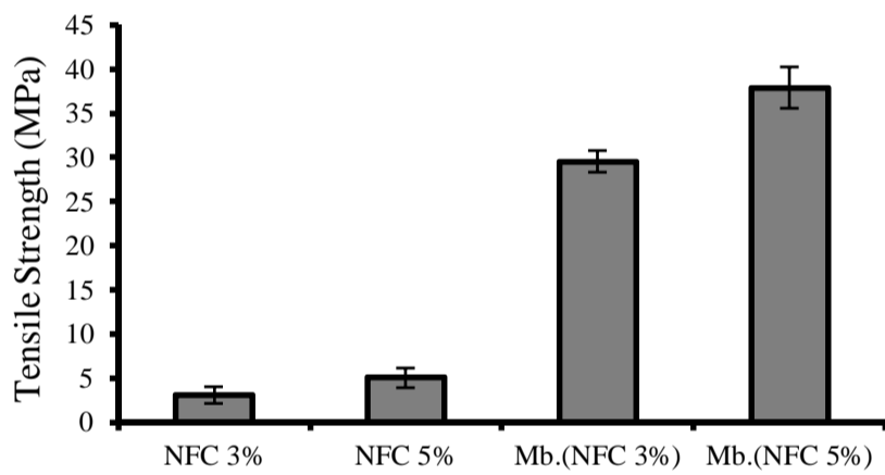
Fig. 8 Comparison tensile strength of nanocomposites with and without masterbatch (NFC: nanocellulose, Mb: masterbatch) شکل 8 مقایسه استحکام کششی نانوکامپوزیت‌های دارای مستریج و بدون آن (NFC: نانوسلولز، Mb: مستریج)
