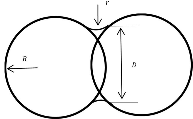
شکل 2 نمایش هندسی نحوه همپوشانی در مکانیزم چسبندگی [10]
