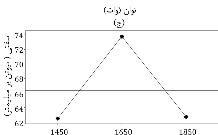
شکل 7 الف-ج تأثیر مستقیم متغیرهای آزمایش بر روی سفتی
