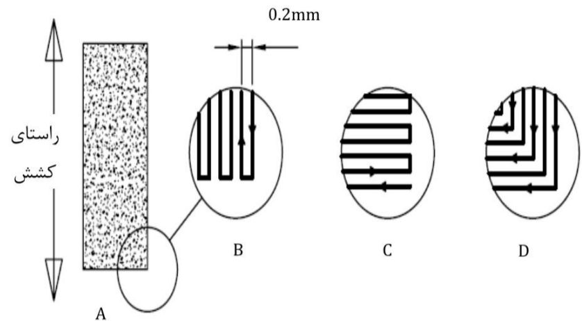
شکل 3 الگوهای مختلف اسکن با فاصله هاشور 0/2 میلیمتر
