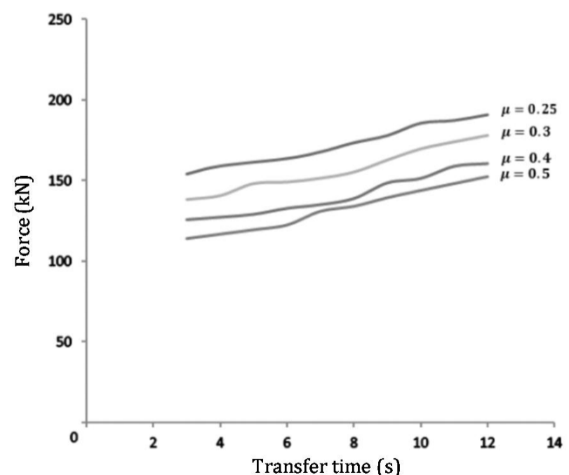
شکل 11 تاثیر اصطکاک در نیروی فرآیند اکستروژن پیش‌فرم پره در آزمایش‌های شبیه‌سازی شده
