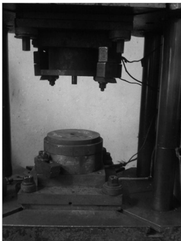
شکل 4 دستگاه پرس اکستروژن
