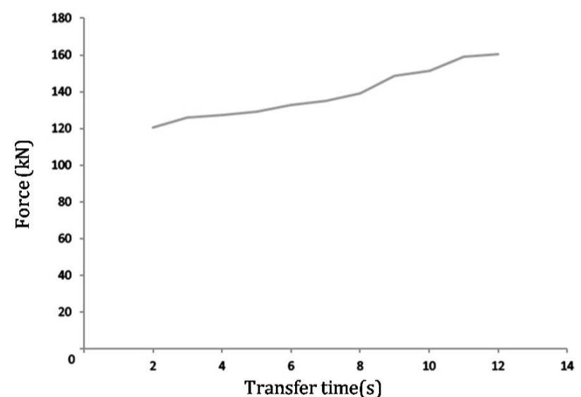
شکل 10 تغییرات نیروی فرآیند با افزایش زمان انتقال در طی آزمایش‌های شبیه‌سازی شده اکستروژن پیش‌فرم پره
