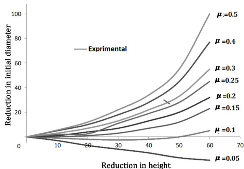
شکل 6 نمودار آزمون فشار حلقه آلیاژ Ti-6Al-4V حاصل از ترکیب نتایج آزمایش‌های شبیه‌سازی و تجربی
