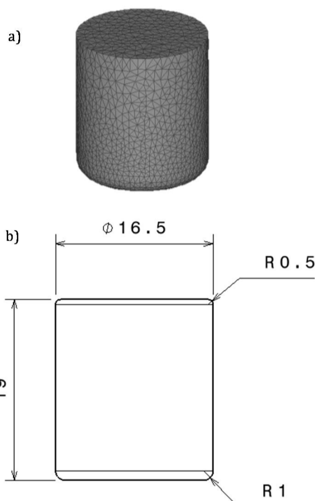
شکل 2 مدل بیلت اولیه (الف) ابعاد هندسی بیلت (ب) ابعاد هندسی بیلت
