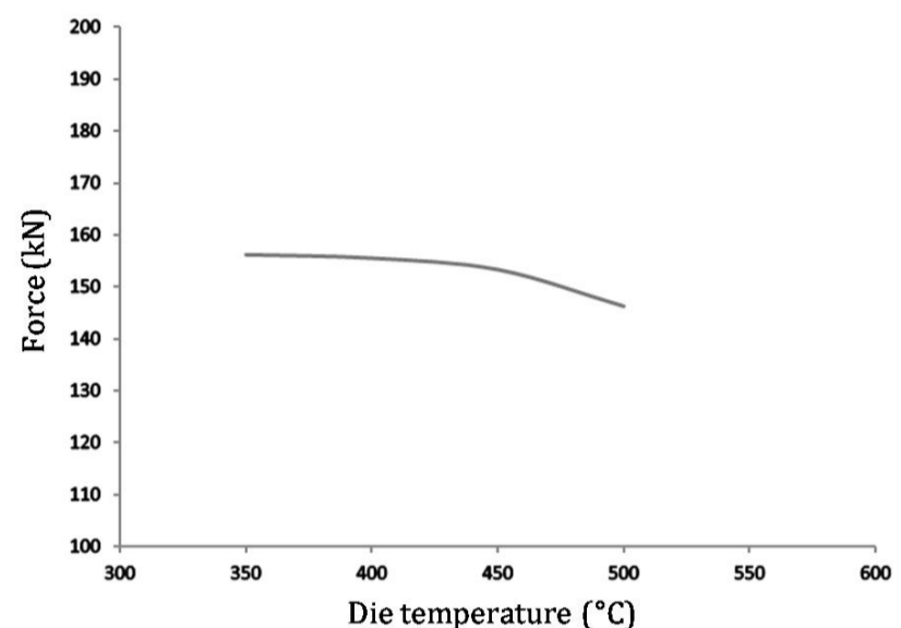
شکل 9 تغییرات نیروی فرآیند نسبت به تغییر دمای قالب در طی آزمایش‌های شبیه‌سازی شده اکستروژن پیش‌فرم پره
