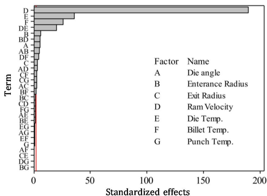
شکل 7 نمودار پارتو حاصل از آزمایش‌های شبیه‌سازی اثرات استاندارد پارامترهای مختلف روی نیروی اکستروژن [1].
