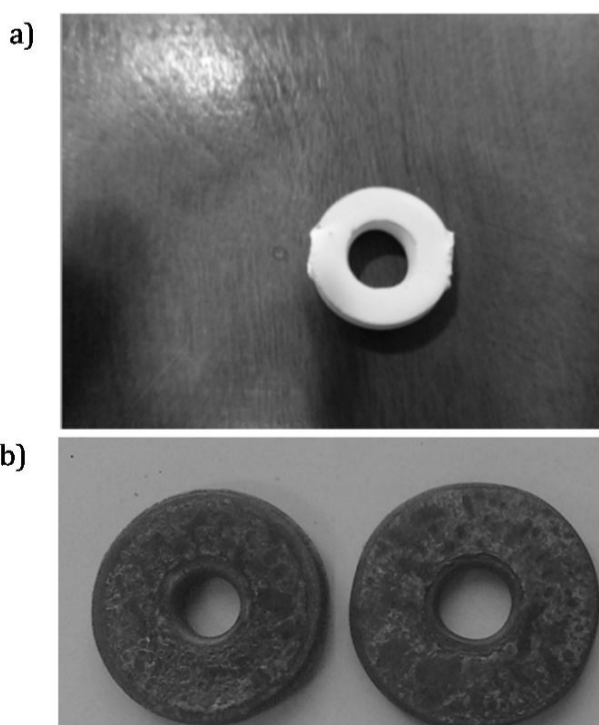
شکل 5 حلقه روان‌کاری شده (الف) قبل از آزمون حلقه (ب) بعد از آزمون حلقه
