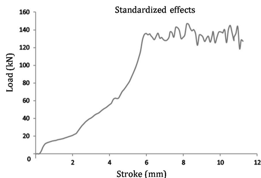
شکل 8 نیروی اکستروژن در طی فرآیند شبیه‌سازی اکستروژن پیش فرم پره آلیاژ Ti-6Al-4V
