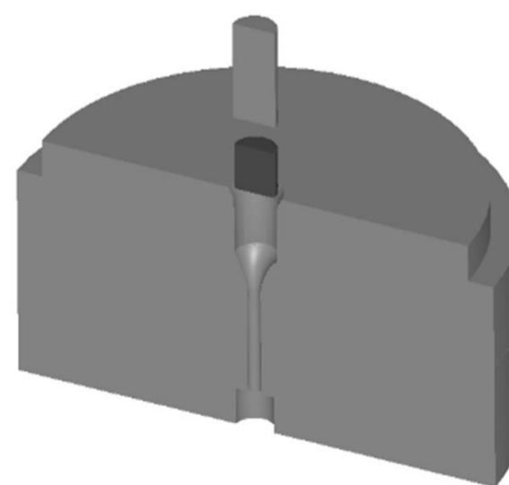
شکل 3 مدل شبیه‌سازی قالب، سنبه و بیلت
