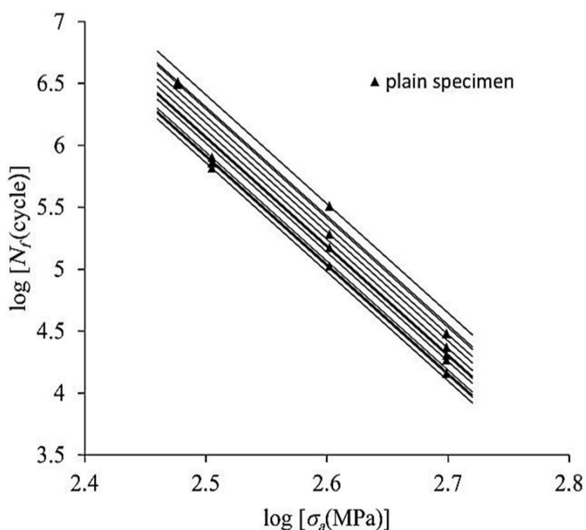
شکل 7 خطوط عبوری از داده‌های خستگی (منحنی‌های عمر تنش در احتمال شکست‌های مختلف)
