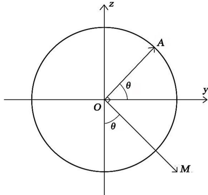
شکل 8 سطح مقطع یک نمونه استوانه‌ای چرخان تحت بارگذاری خمشی
