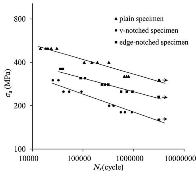
شکل 6 نمودار تنش عمر سه نمونه آزمایش شده در مقیاس لگاریتمی
