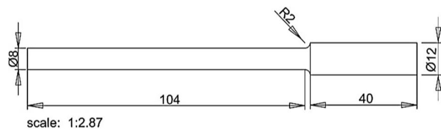
شکل 2 جزئیات ابعاد نمونه با فاق پله‌ای برای آزمایش خستگی
