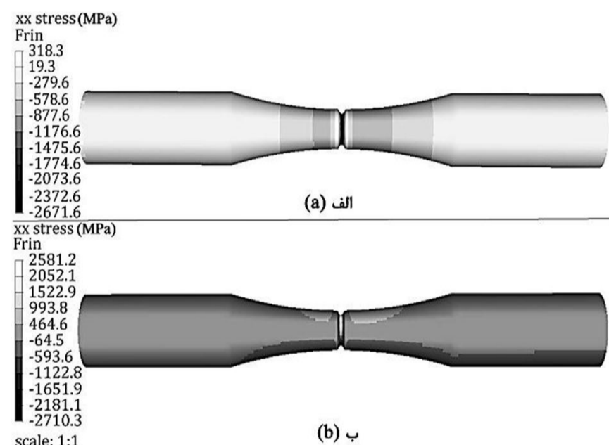
شکل 9 تفاوت توزیع تنش در دو حالت چرخان (الف) و استاتیکی (ب) برای نمونه با فاق 7 شکل
