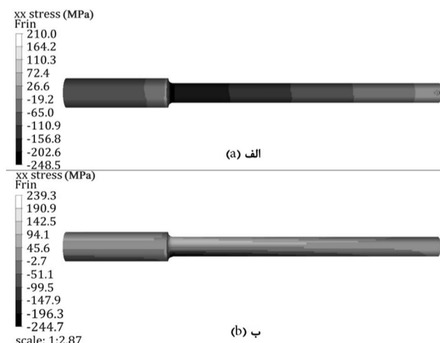
شکل 10 تفاوت توزیع تنش در دو حالت چرخان (الف) و استاتیکی (ب) برای نمونه با فاق پله‌ای
