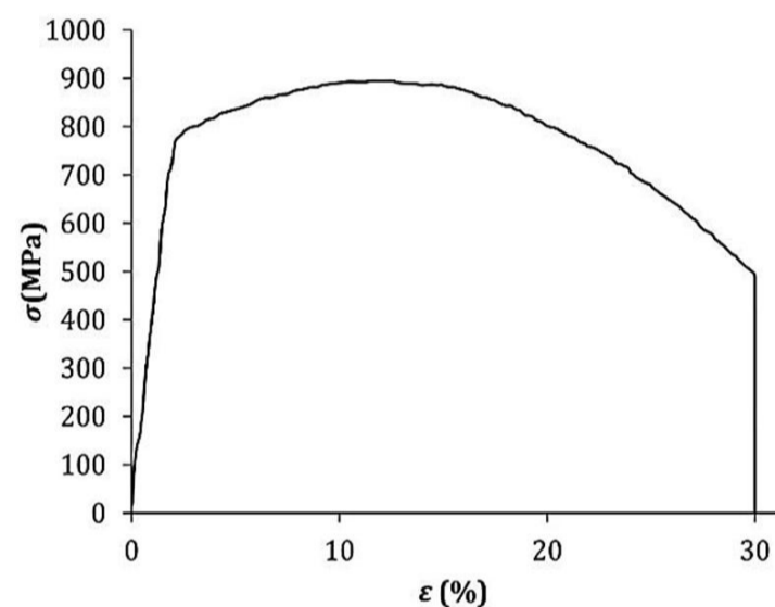
شکل 1 نمودار تنش - کرنش فولاد HSLA100
