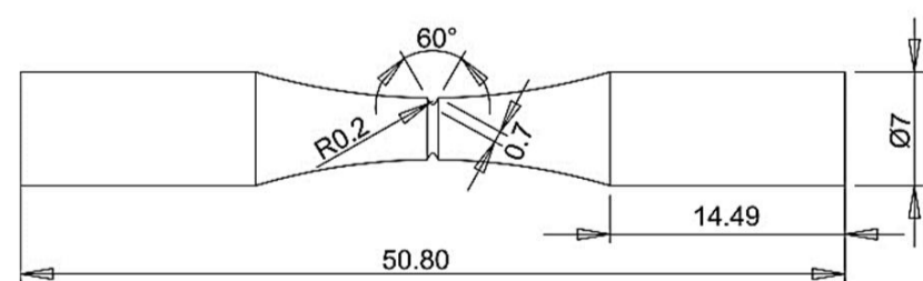
شکل 3 جزئیات ابعاد نمونه ساده و نمونه با فاق V شکل برای آزمایش خستگی
