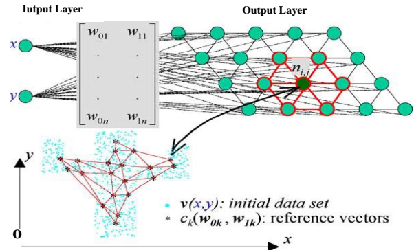
شکل ۱- ساختار یک نگاشت خودسازمانده (۴×۵)
