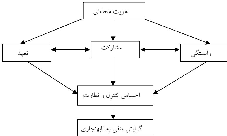
شکل ۱. الگوی تحقیق
