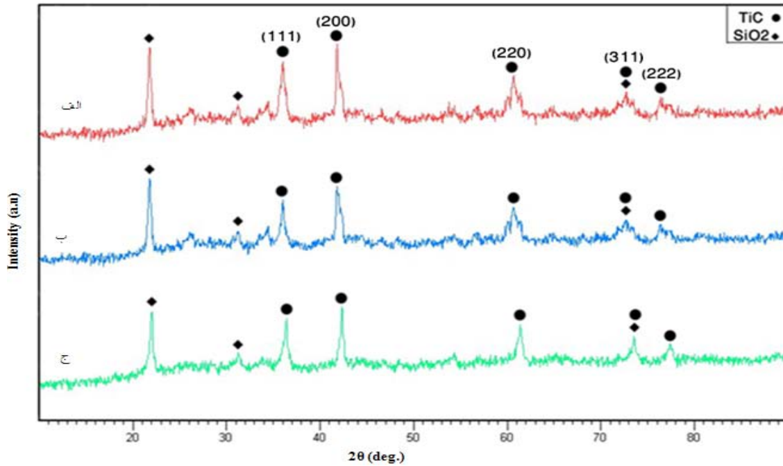
شکل (۵): الگوی پراش اشعه ایکس نمونه‌های (الف): ۱۰ ساعت آسیاب کاری شده و سنتز در دمای 1200^{\circ}C ، (ب): ۲۰ ساعت آسیاب کاری شده و سنتز در دمای 1000^{\circ}C و (ج): ۶۰ ساعت آسیاب کاری شده و سنتز در دمای 900^{\circ}C .
