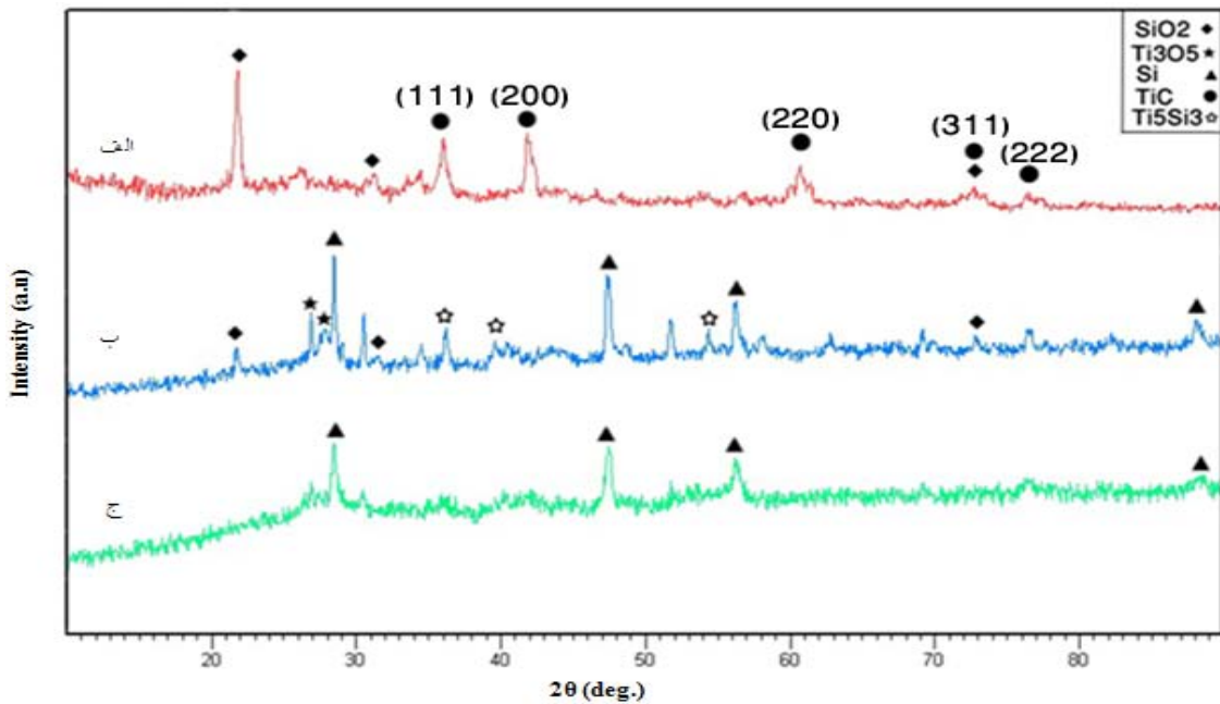
شکل (۴): الگوی پراش اشعه ایکس نمونه‌های (الف): ۱۰ ساعت آسیاب کاری شده و سنتز در دمای 1200^{\circ}\text{C} ، (ب): ۲۰ ساعت آسیاب کاری شده و سنتز در دمای 950^{\circ}\text{C} و (ج): ۶۰ ساعت آسیاب کاری شده و سنتز در دمای 800^{\circ}\text{C}
