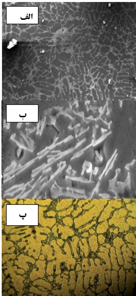
شکل (۲): ریزساختار نمونه‌های ریخته‌گری شده در دمای 75^{\circ}\text{C} با اندازه ذرات 300\ \mu\text{m} : (الف) تصویر SEM با بزرگنمایی 200\times ، (ب) تصویر SEM با بزرگنمایی 200\times و (پ) تصویر میکروسکوپ نوری با بزرگنمایی 400\times
