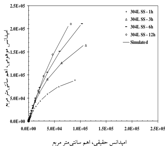
شکل (۱۱): منحنی نایکویست و مدل‌سازی شده با استفاده از مدار معادل شکل ۱۰ برای فولاد زنگ‌نزن ۳۰۴ کم کربن در محلول شبیه‌سازی بتن.
