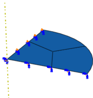
شکل (۴): شرایط مرزی اعمال شده بر ورق
