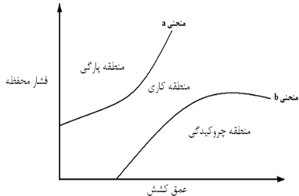
شکل (۲): محدوده فشار کاری در فرآیند هیدروفورمینگ
