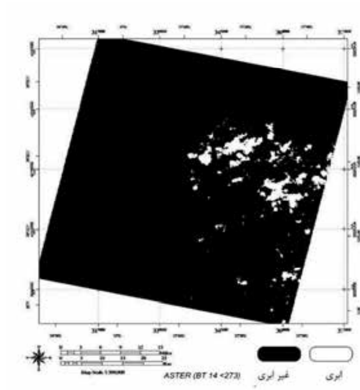
شکل ۵ نتیجه حاصل از آستانه گذاری تصویر BT ۱۴
