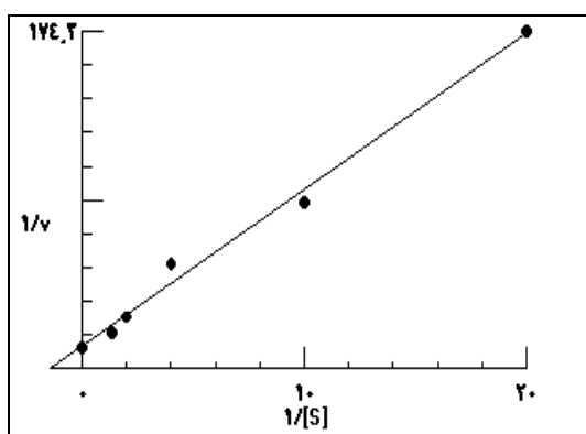
شکل ۵. منحنی لاینویور- بارک برازش شده برای آلفا-آمیلاز لارو سن سوم کفشدوزک خربزه
