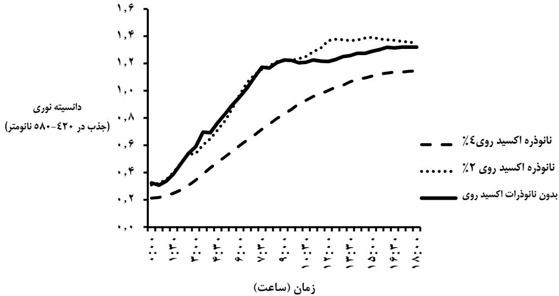
شکل ۳- منحنی رشد باکتری باسیلوس سویبتیلیس در حضور و عدم حضور نانوذرات اکسید روی
