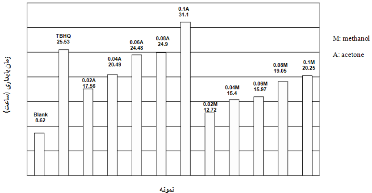
نمودار ۱- زمان پایداری در برابر اکسیداسیون تیمارهای مختلف تالو در دمای ۱۱۰ درجه سانتی‌گراد
