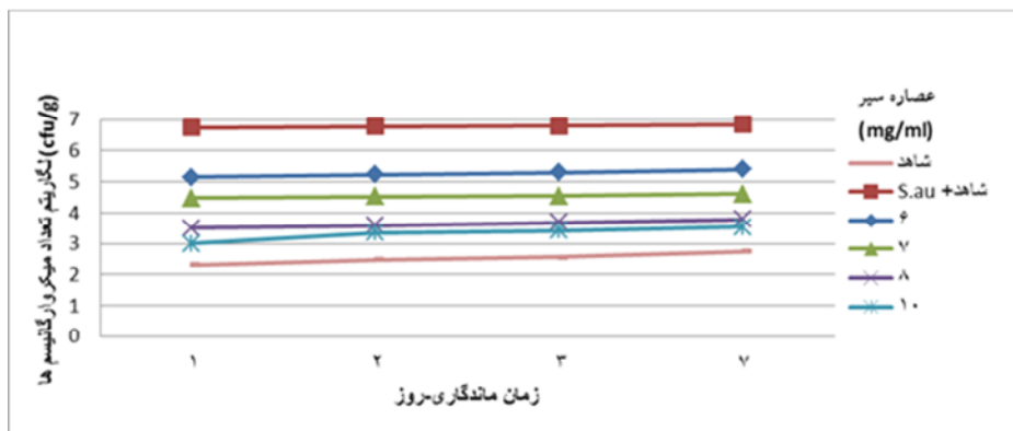
نمودار ۲- اثر غلظت‌های مختلف عصاره سیر بر شمار باکتری S. aureus در گوشت مرغ آماده طبخ در درجه حرارت ۴ درجه سانتی‌گراد
