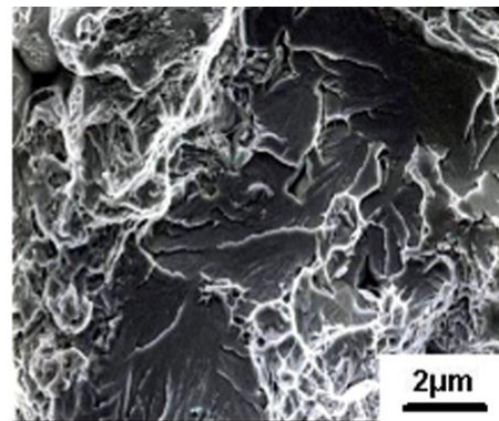
شکل ۳- ریز ترک مشاهده شده در ساختار فولاد D.HP و توقف آن در ناحیه آستنیت در بزرگنمایی کم (الف) و زیاد (ب).
