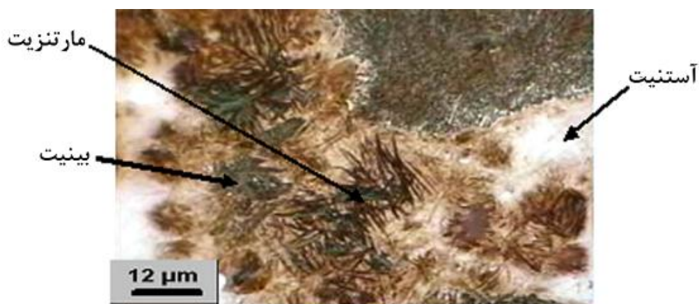
شکل ۲- ریزساختار عمومی فولاد HP.
