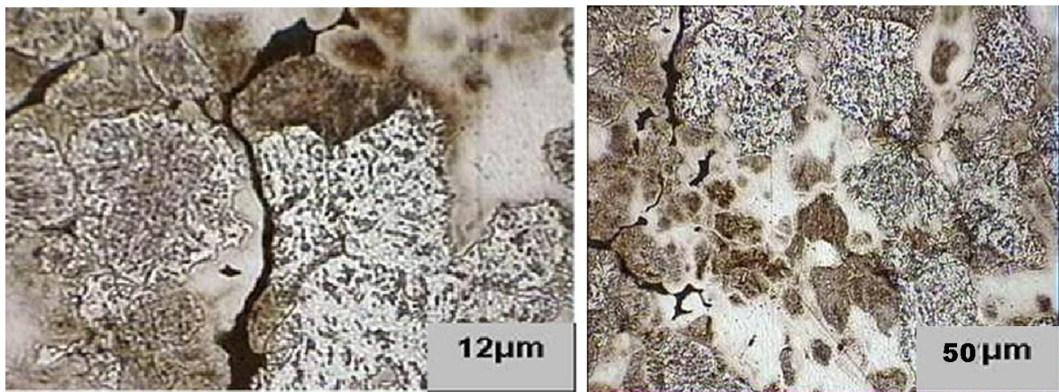
شکل ۳- ریز ترک مشاهده شده در ساختار فولاد D.HP و توقف آن در ناحیه آستنیت در بزرگنمایی کم (الف) و زیاد (ب).
