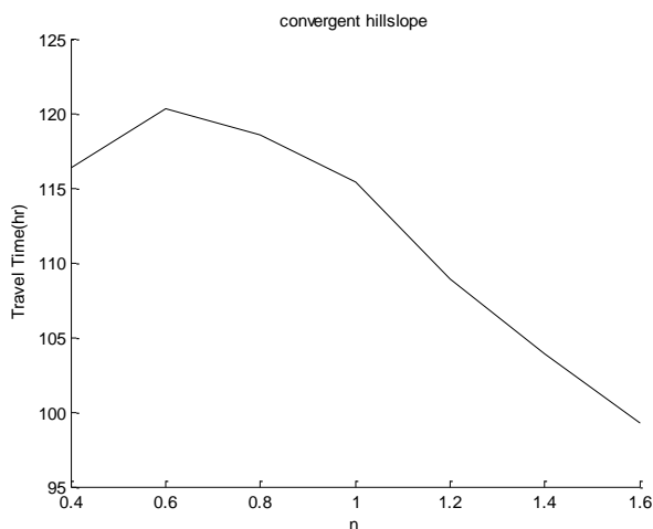
شکل ۸- اثر تغییرات میزان انحنا برای دامنه‌های همگرا (N=50mm/day)
