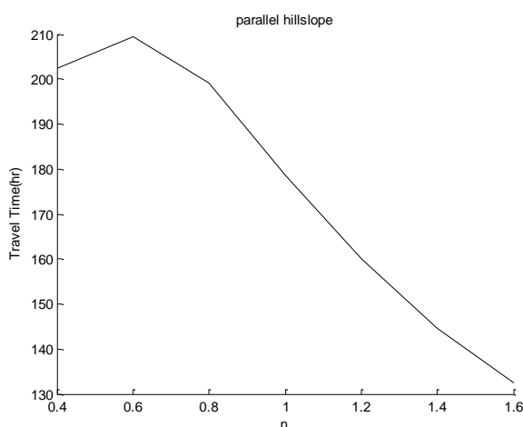
شکل ۷- اثر تغییرات میزان انحنا برای دامنه‌های موازی (N=50mm/day)
