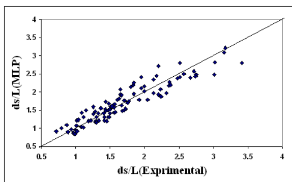
شکل ۴- مقایسه‌ی ds/l محاسبه‌شده با کاربرد روش MLP و داده‌های آزمایشگاهی برای آبشکن بالدار.
