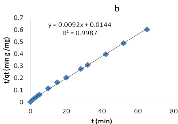
شکل ۷- شبیه جنبشی شبه درجه‌ی اول (a) و شبه درجه‌ی دوم (b) جذب رنگ بازی فوشین به‌وسیله‌ی سبوس برنج.
