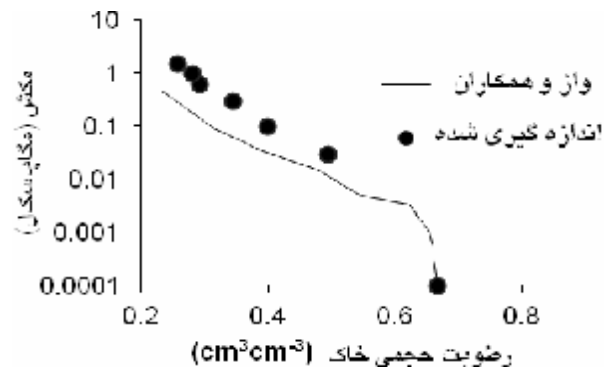
شکل 3- برآورد منحنی مشخصه آب خاک در خاک رس سیلتی (خاک شماره 2) با استفاده از \alpha از واز و همکاران (2005) در مدل آریا و پاریس
