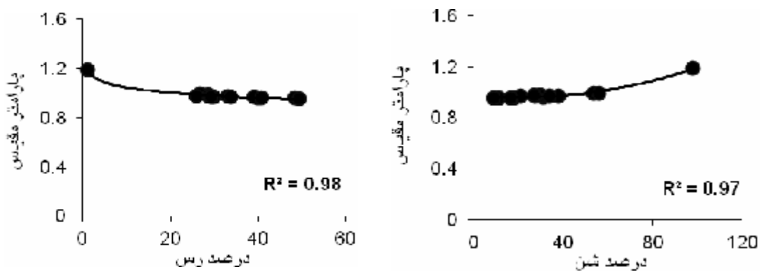
شکل 4- نمودار رابطه درصد رطوبت خاک با پارامتر مقیاس پیشنهادی واز و همکاران (2005) در 14 خاک مورد مطالعه
