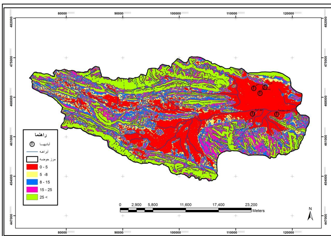
شکل ۴. نقشه شیب حوضه شور فدای
