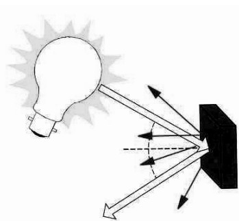
شکل ۱: برخورد نور با یک جسم پشت‌پوش [۳].
