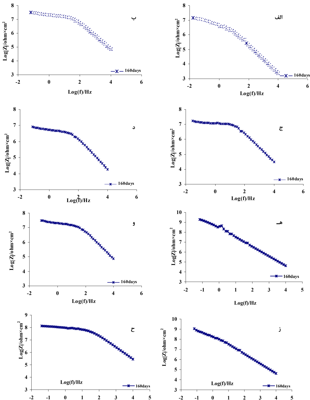
شکل ۸: نمودارهای بد مربوط به نمونه‌های نانوکامپوزیت اپوکسی، الف) پلی آمیدوآمین ۱/C30B، ب) سیکلوالیفاتیک آمین ۱/C30B، ج) پلی آمیدوآمین ۲/C30B، د) سیکلوالیفاتیک آمین ۲/C30B، ه) پلی آمیدوآمین ۳/C30B، و) سیکلوالیفاتیک آمین ۳/C30B، ز) پلی آمیدوآمین ۴/C30B و ح) سیکلوالیفاتیک آمین ۴/C30B پس از ۱۶۰ روز غوطه‌وری در محلول ۳،۵ درصد کلریدسدیم.
