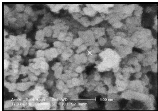
کمپلکس نیکل ۲۵٪
