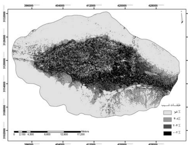
شکل ۴- نقشه شیب
