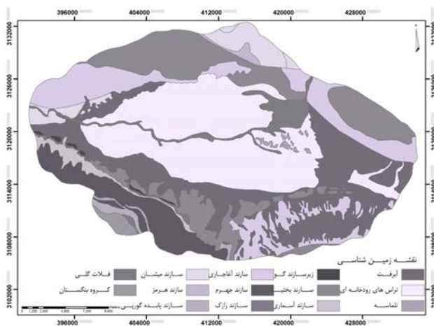
شکل ۶- نقشه زمین‌شناسی
