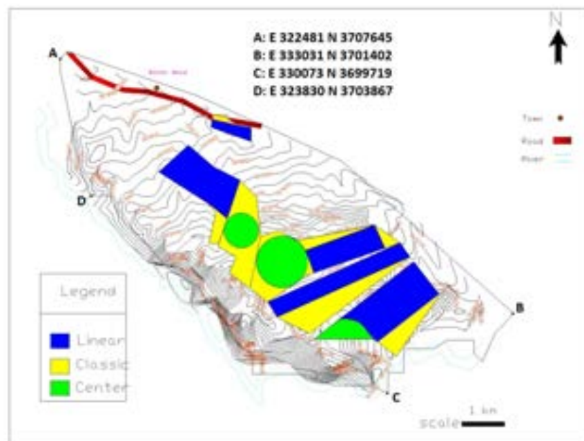
شکل ۷ - نقشه جانمایی انواع سیستم‌های آبیاری (نقشه شماتیک انواع سیستم‌های آبیاری)
