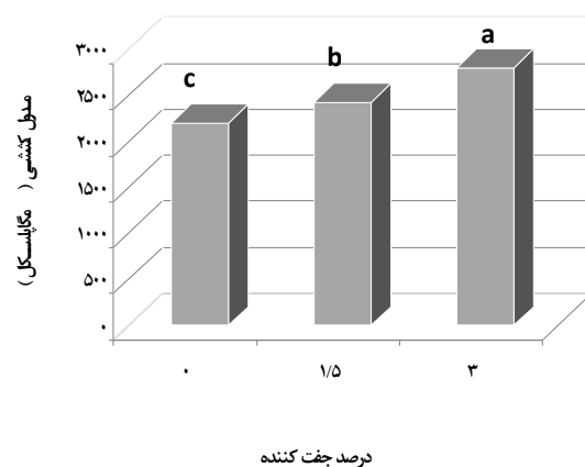
شکل 2 - اثر مستقل درصد جفت کننده بر مقاومت و مدول کششی چندسازه چوب پلاستیک
