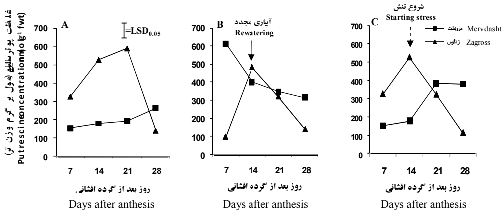
شکل ۱- تغییرات غلظت پوترسین دانه‌های در حال رشد ارقام گندم زاگرس و مرودشت در مراحل مختلف رشد دانه در رژیم‌های خشکی پس از گرده‌افشانی. الف: شاهد، ب: تنش از ۵۰ درصد گرده‌افشانی تا ۱۴ روز بعد و ج: تنش خشکی از ۱۴ روز بعد از گرده‌افشانی تا پایان دوره رشد. I: شاخص تفاوت معنی‌داری LSD در سطح پنج درصد
