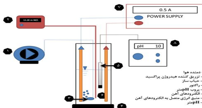
شکل ۱- تصویر شماتیک سیستم مورد استفاده در فرآیند الکتروفنتون
