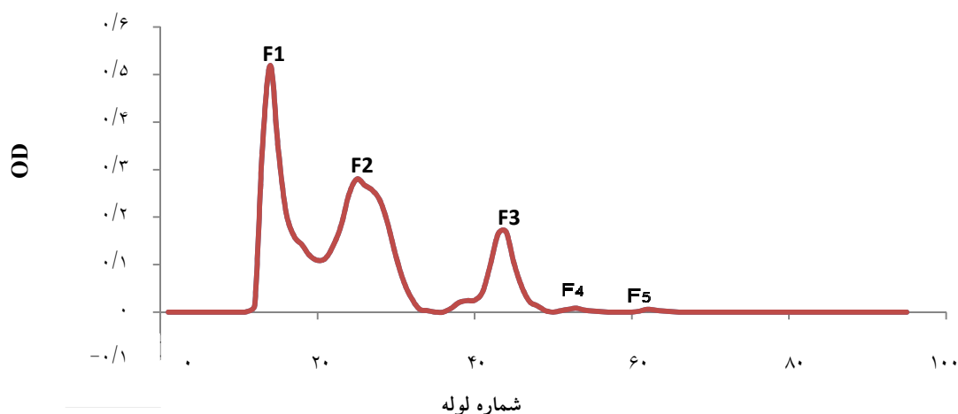
نمودار ۱: ژل کروماتوگرافی 50 mg زهر خام با استفاده از سفادکس G-75
