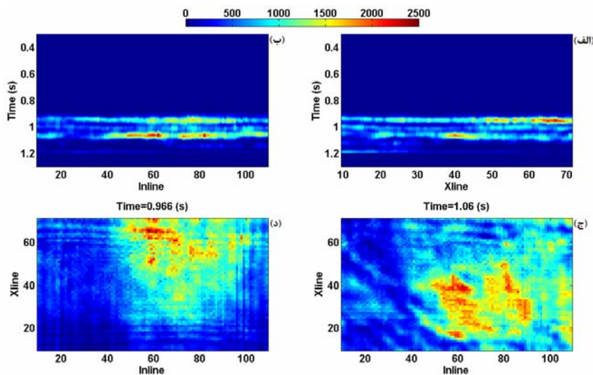
شکل ۱۲. برش قائم از مکعب شکل (۶ چپ) در راستای الف) خط گیرنده ۴۱، ب) خط چشمه ۴۱ و برش افقی در راستای ج) زمان 1/060 ثانیه و د) زمان 0/966 ثانیه.
