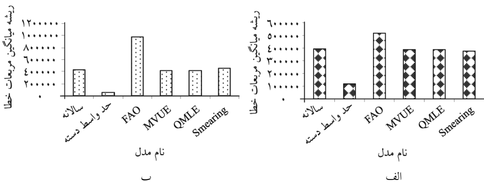
شکل ۴- هیستوگرام مقادیر شاخص آماری ریشه میانگین مربعات خطا (RMSE) برای مدل ۸۰-۲۰ (الف) و تمام داده‌ها (ب).
