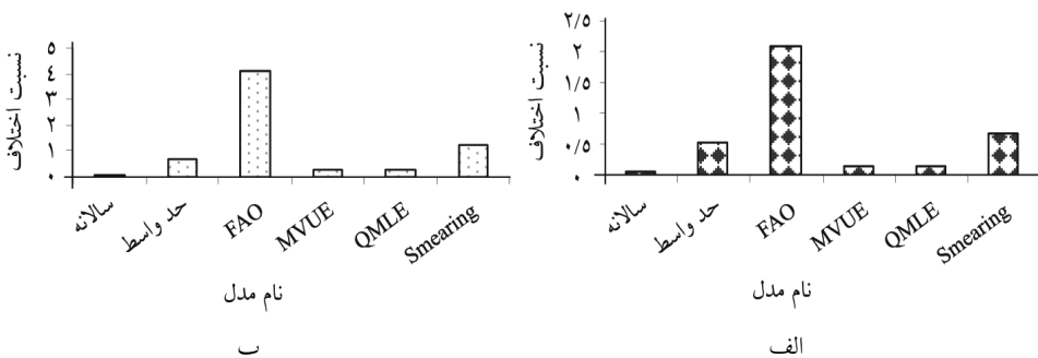
شکل ۳- هیستوگرام مقادیر شاخص آماری نسبت اختلاف (RV) برای مدل ۸۰-۲۰ (الف) و تمام داده‌ها (ب).
