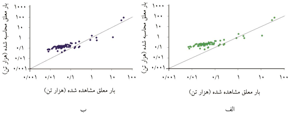
شکل ۵- مقایسه مقادیر بار معلق مشاهده شده و محاسبه شده برای مدل ۸۰-۲۰ (الف) و تمام داده‌ها (ب).
