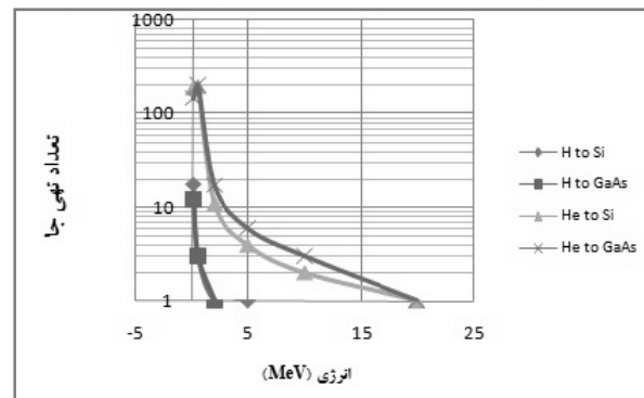
شکل ۲- تهی جا ناشی از پرتوی ورودی یون هیدروژن و هلیوم در قطعات الکترونیکی
