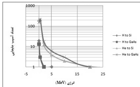
شکل ۱- آسیب جابه‌جایی ناشی از پرتوی ورودی یون هیدروژن و هلیوم در قطعات الکترونیکی
