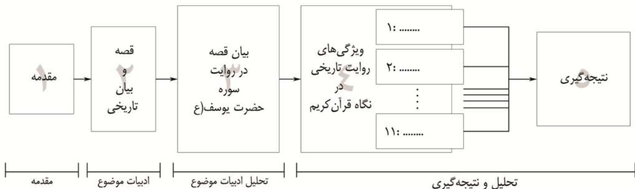
شکل ۱: الگوی تحقیق
