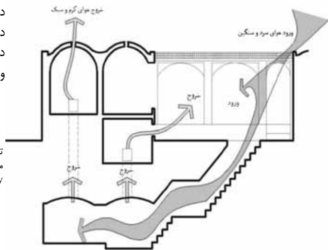
تصویر ۲. برش عمودی از شوادون و چگونگی خروج و ورود هوا. مأخذ : بینا، ۱۳۸۷.
