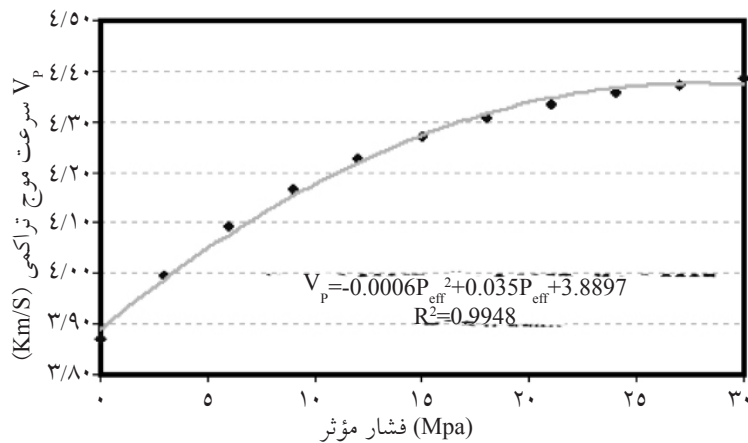
شکل ۴- تغییر سرعت موج V_p در اثر تغییرات فشار مؤثر
