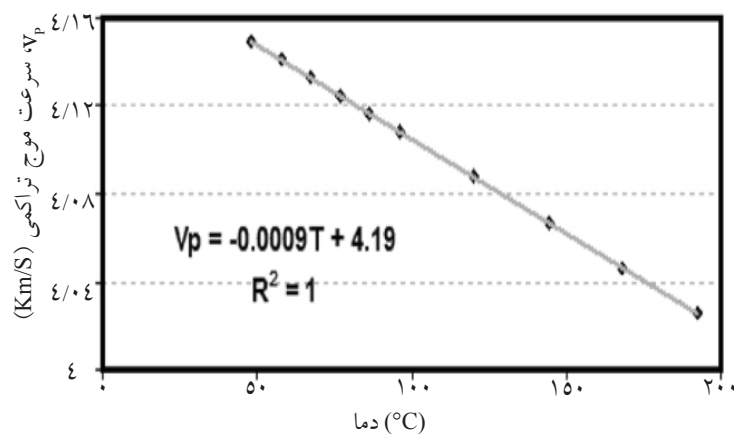
شکل ۶- تغییر سرعت موج V_p در اثر تغییر درجه حرارت
